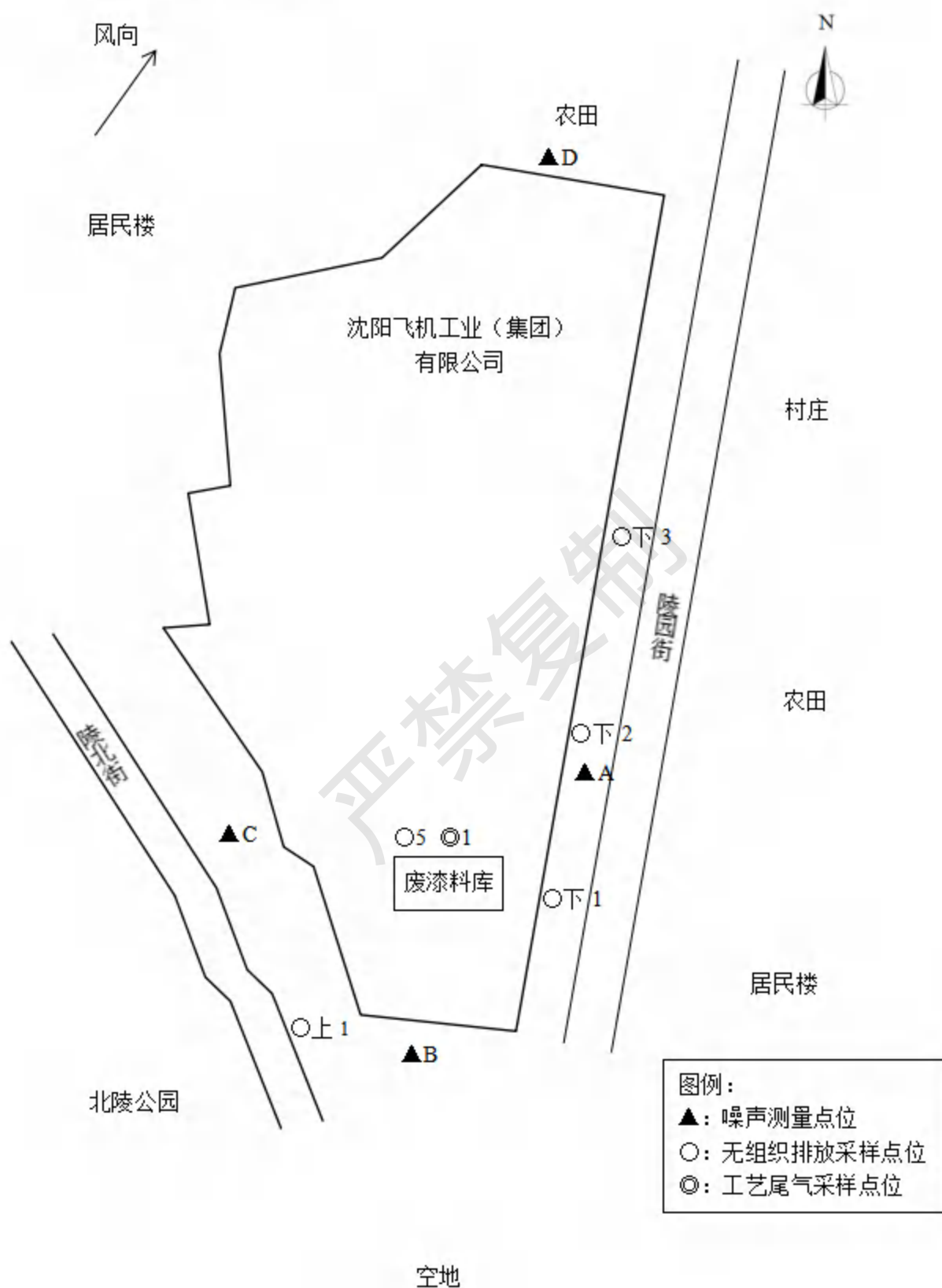
图 7-1 试飞站废漆料库改造项目监测点位示意图
