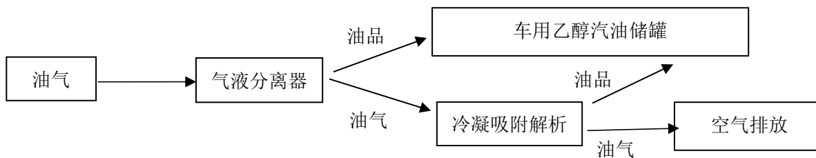
图 2-6 三次油气回收工艺流程框图
