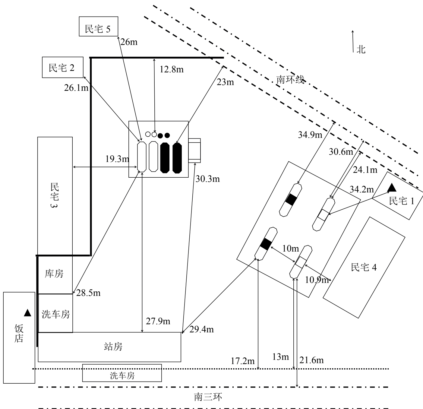
图 2-1 周边环境及总平面布置图
