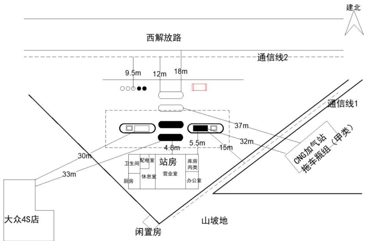
图 2.3-1 周边环境及总平面布置图
