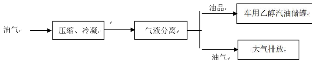
图 2.6-5 三次油气回收工艺流程框图
