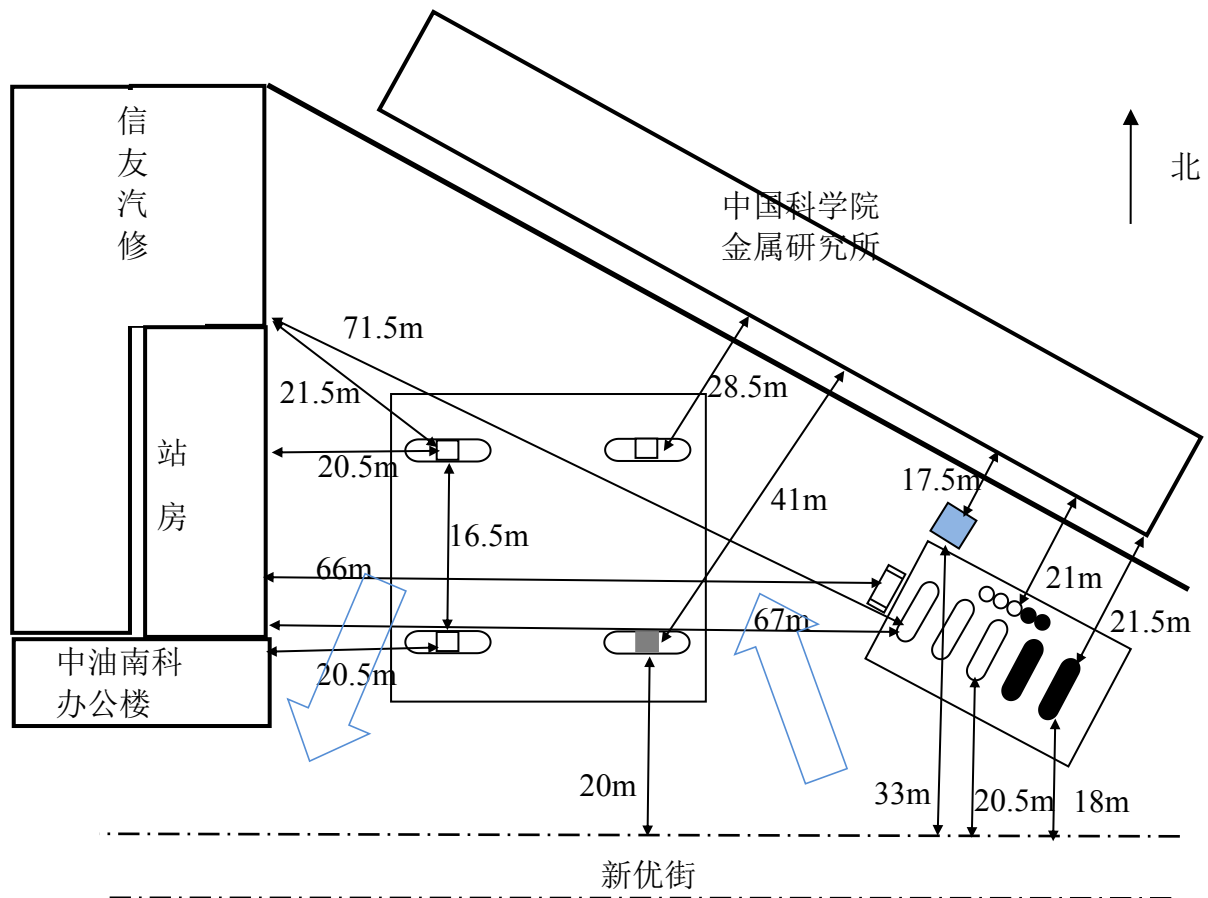
图 2.3-1 周边环境及总平面布置图
