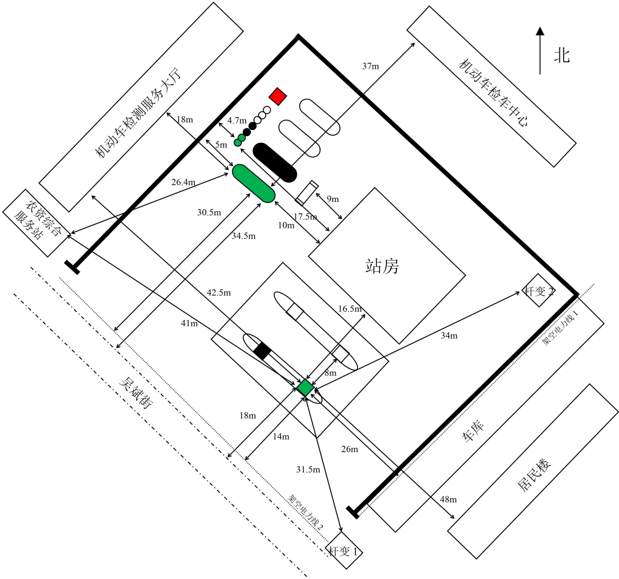
图 2-1 周边环境及总平面布置图
