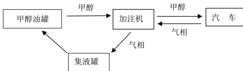
图 2.5-2 加注及加注气相回收工艺流程图
