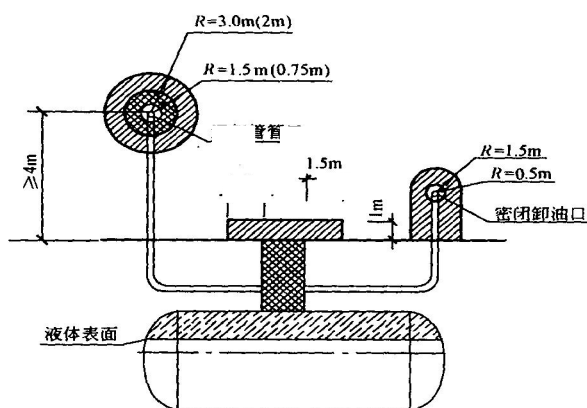
图 3 埋地卧式汽油储罐爆炸危险区域划分图
