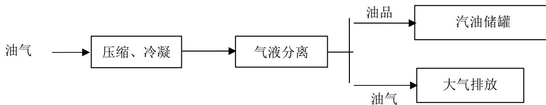
图 2-6 汽油三次油气回收工艺流程框图
