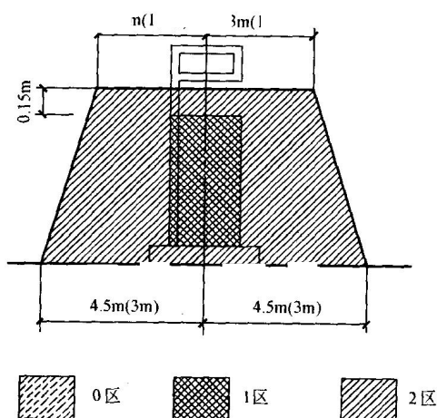
图 1 汽油加油机爆炸危险区域划分
