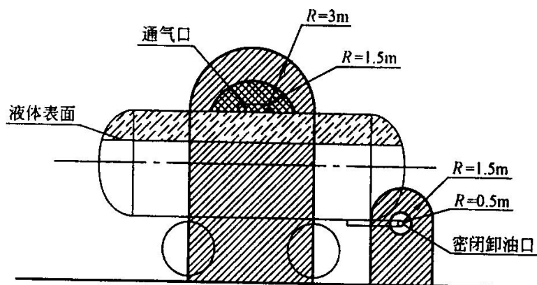
图 2 油罐车卸汽油时爆炸危险区域划分
